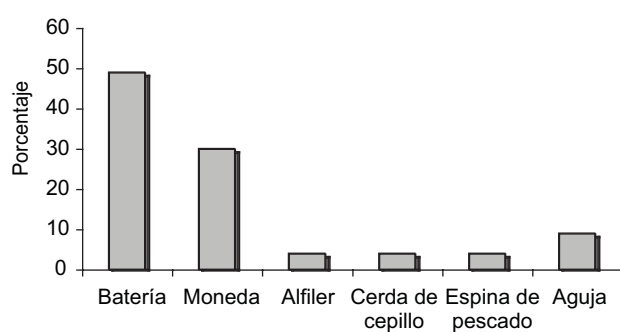
Figura 11. Objeto injerido.
