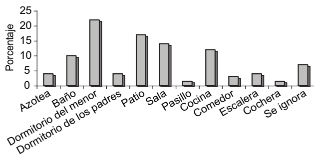
Figura 4. Lugar.
