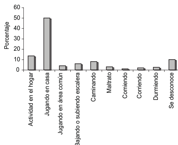
Figura 10. Circunstancia.
