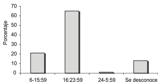
Figura 9. Hora.
