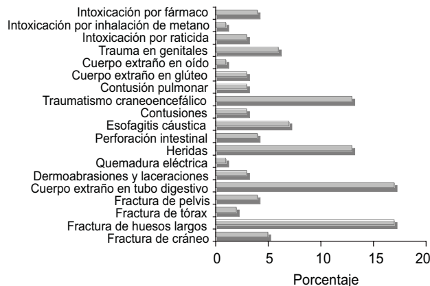
Figura 6. Diagnóstico.
