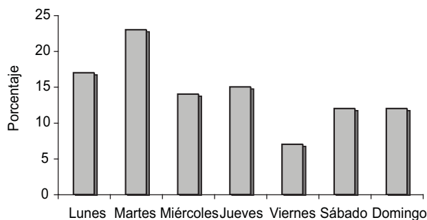
Figura 8. Día.
