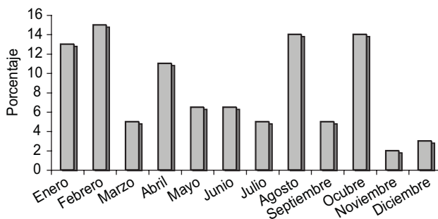
Figura 7. Mes.
