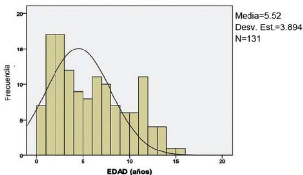
Figura 1. Histograma.
